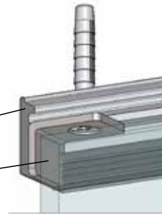
PORTA CON CERNIERE VETRO-VETRO (IL PESO DELLA PORTA GRAVA SUL FISSO) PUERTA CON BISAGRA VIDRIO-VIDRIO (EL PESO DE LA PUERTA SOBRE EL VIDRIO FIJO) DOOR WITH GLASS-GLASS HINGES (The door weight is beard on the fixed panel) GLAS-GLAS BÄNDER (Befestigung an Seitenteil)
